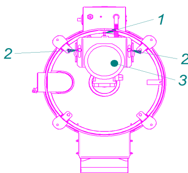
Рисунок 4. Натяжение ремня
