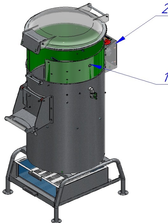
Рис.3. Абразив боковой
