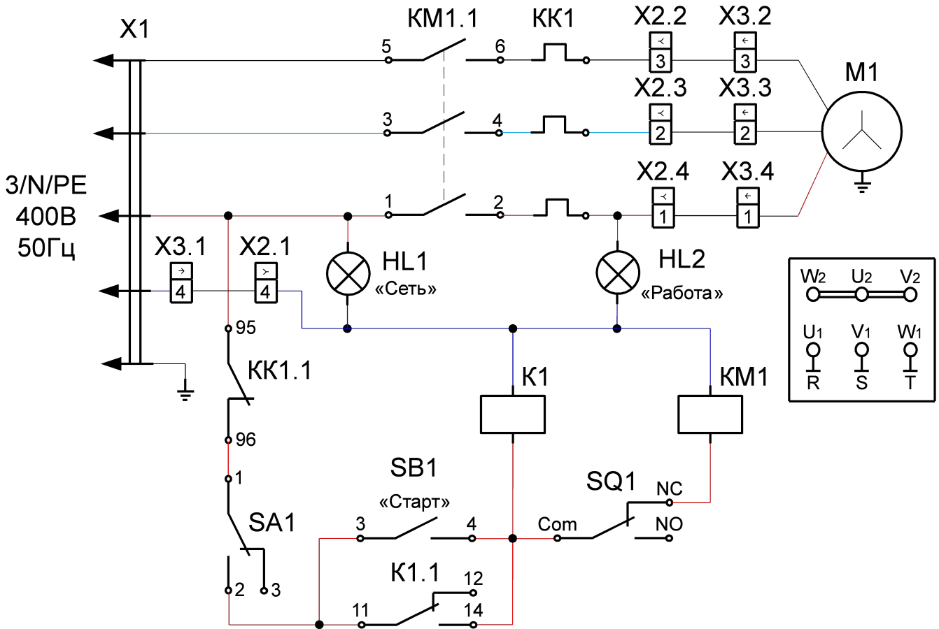
СХЕМА ЭЛЕКТРИЧЕСКАЯ ПРИНЦИПАЛЬНАЯ МКК-150, МКК-300
